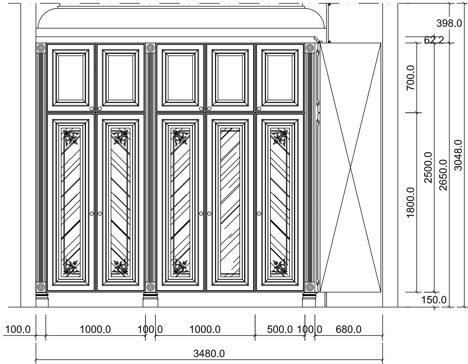
ELEVATION A
