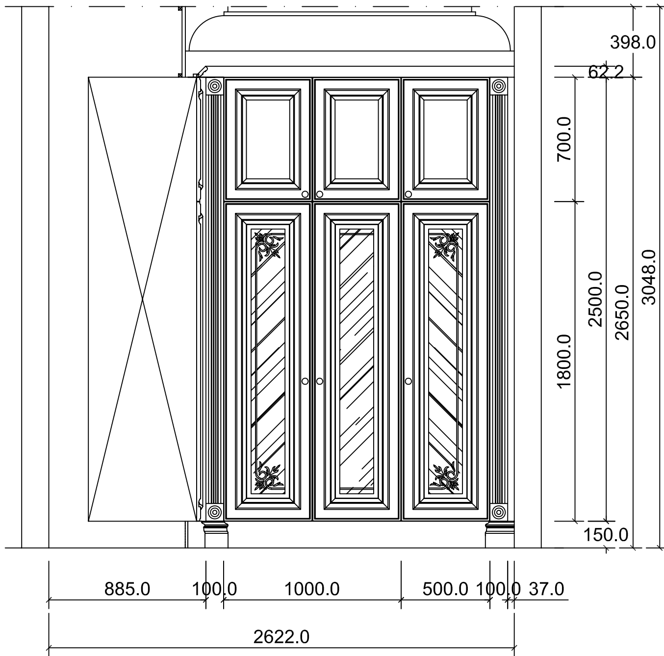
ELEVATION B
