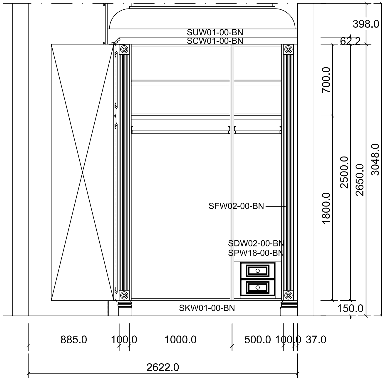
ELEVATION B
