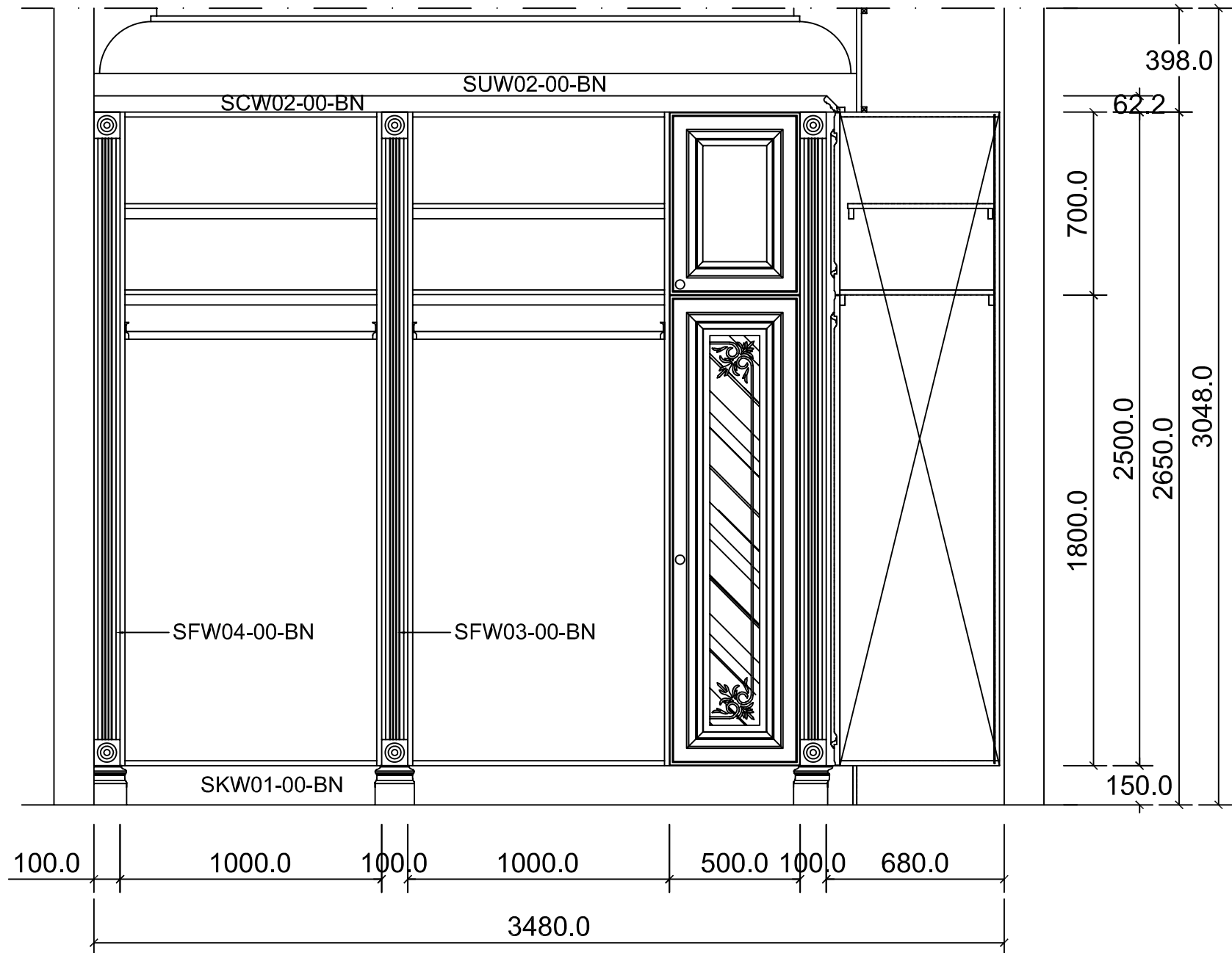
ELEVATION A
